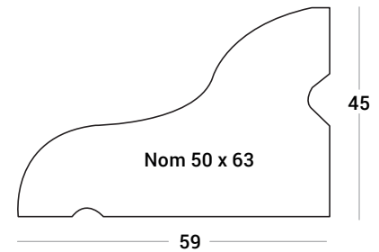
Door Drip
