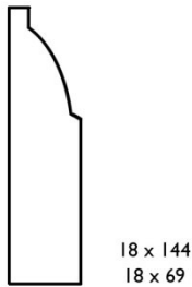
Ovolo
